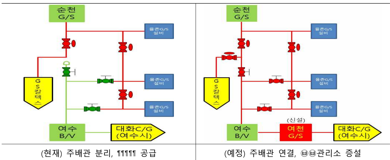
【그림 4】 ㉑㉒GS 주배관 분리 및 연결 계통도
