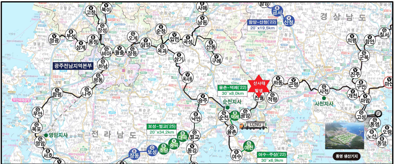
【그림 1】㉔㉕관리소 위치 및 가스공급 배관망도
